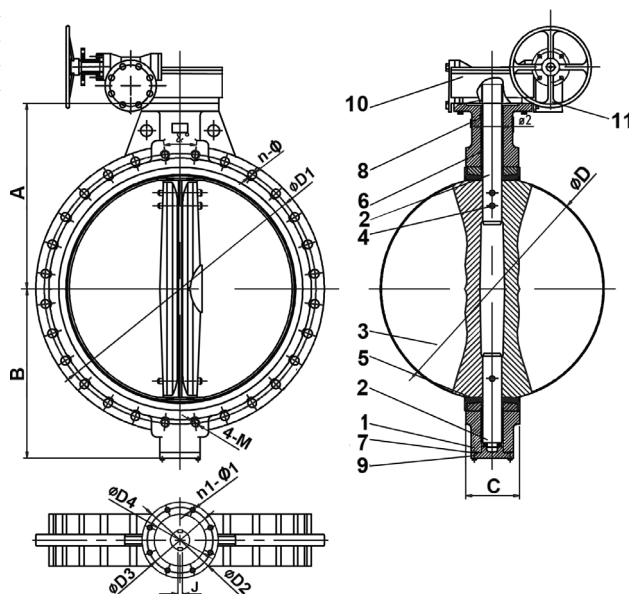
DN700 - DN1200
